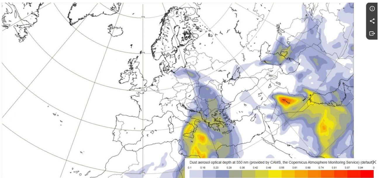
Evoluția masei de aer încărcate cu particule de praf 16 aprilie, ora 6
