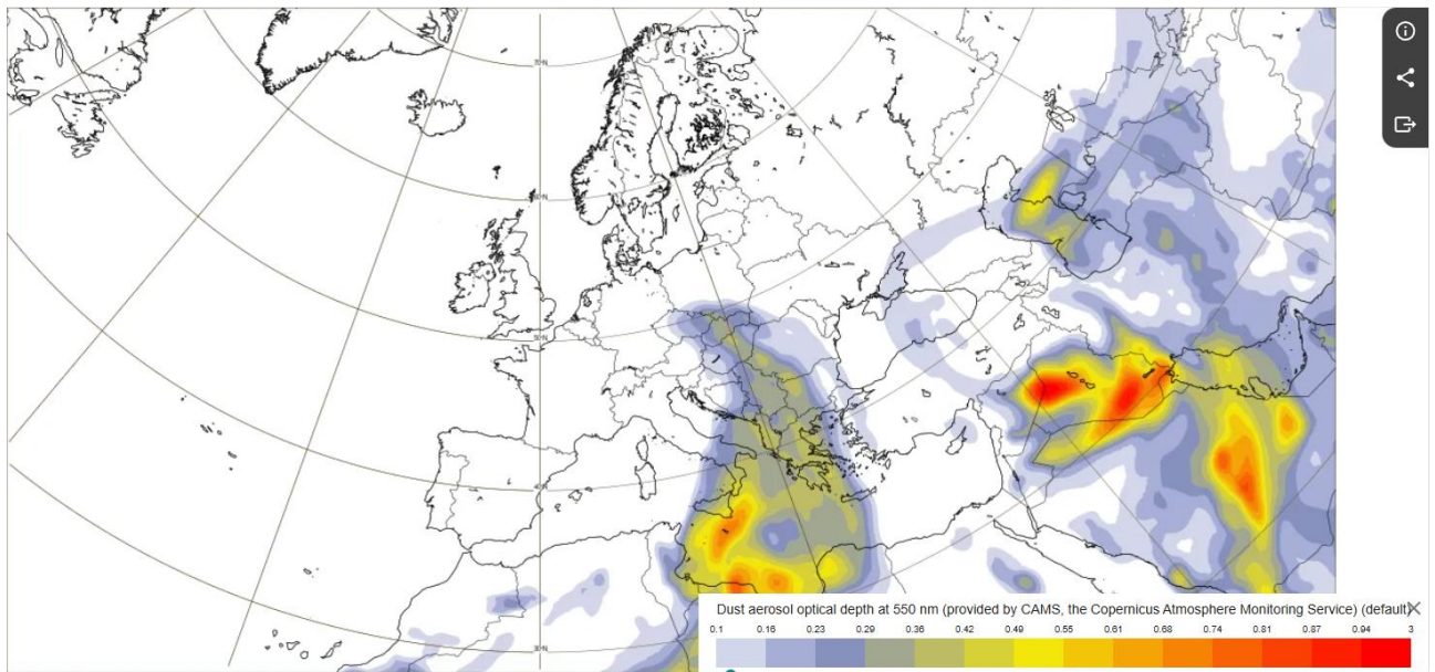
Evoluția masei de aer încărcate cu particule de praf 15 aprilie, ora 21
