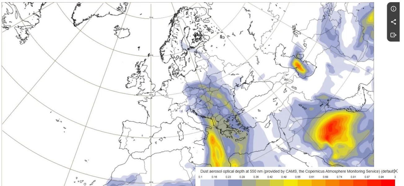
Evoluția masei de aer încărcate cu particule de praf 17 aprilie, ora 6
