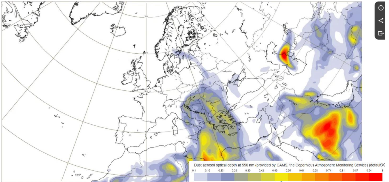
Evoluția masei de aer încărcate cu particule de praf 16 aprilie, ora 21
