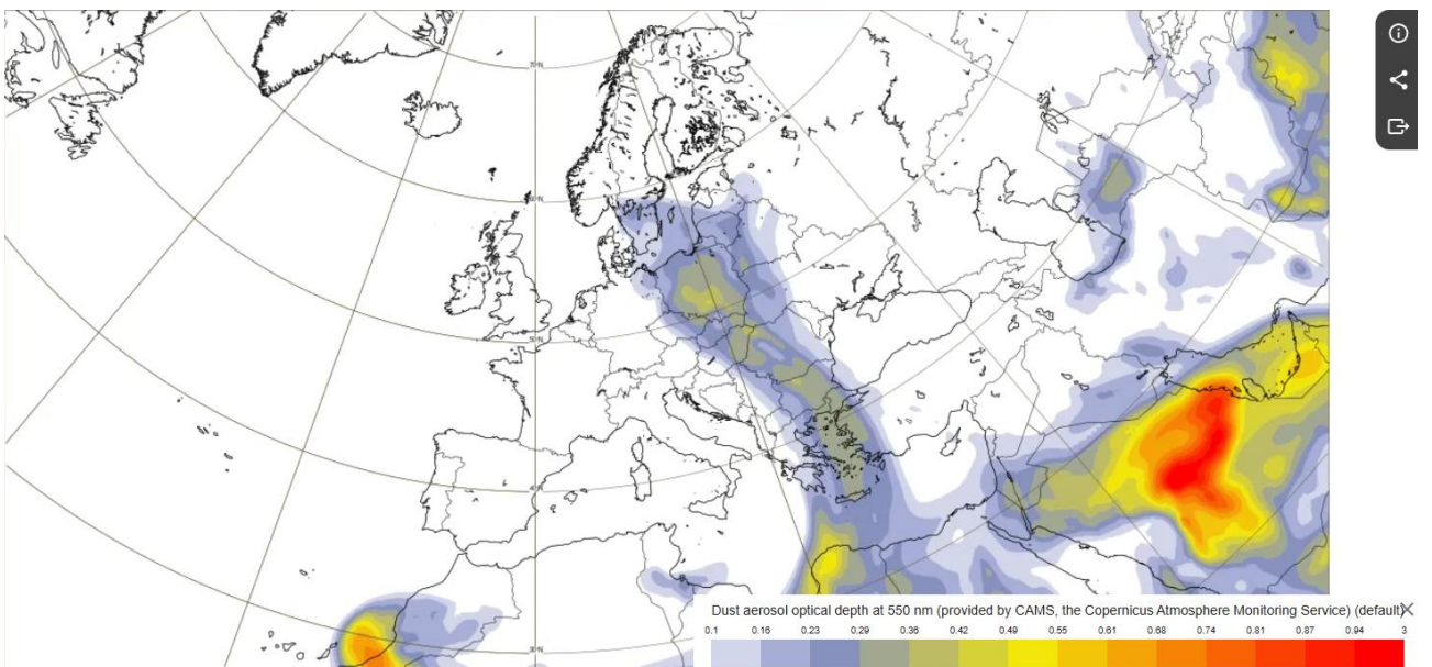
Evoluția masei de aer încărcate cu particule de praf 18 aprilie, ora 3
