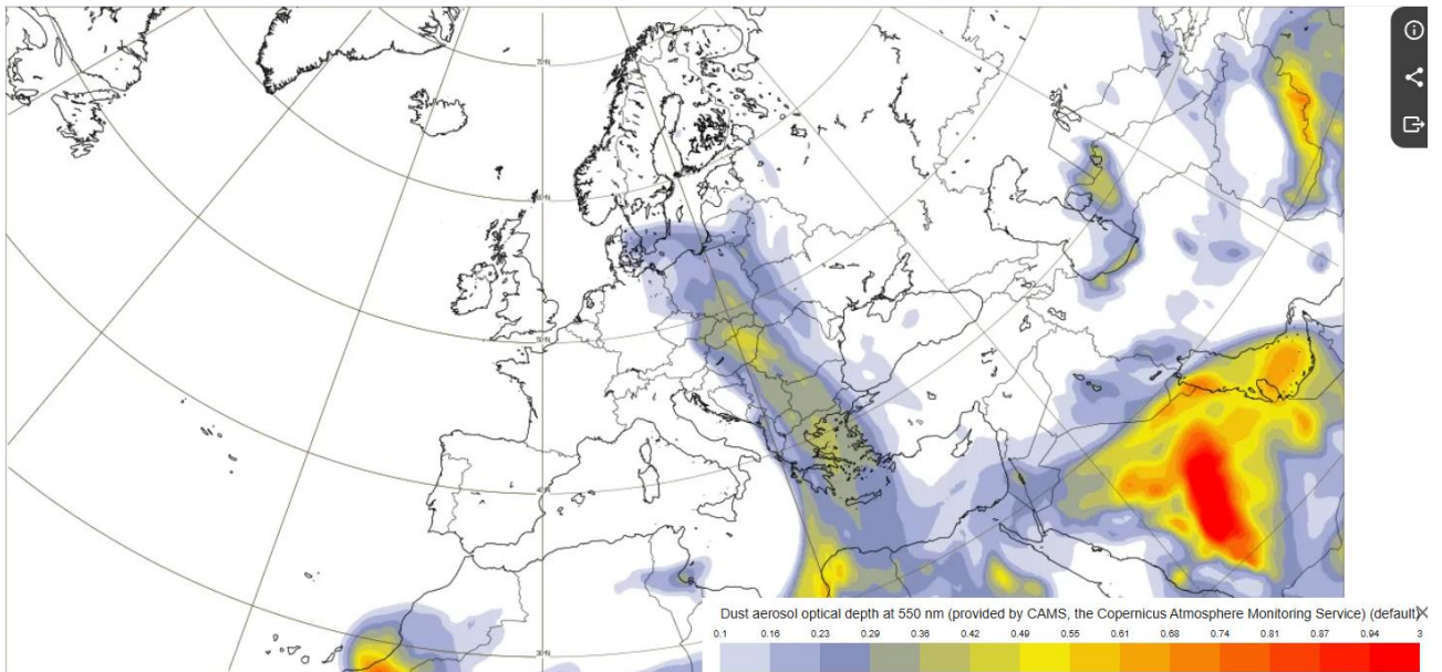
Evoluția masei de aer încărcate cu particule de praf 17 aprilie, ora 21
